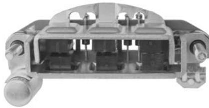
131221 Rectifier
