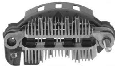
236559 Rectifier
