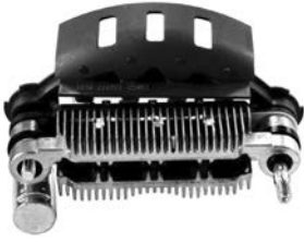
136977 Rectifier
