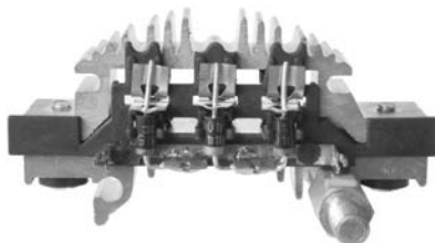
132673 Rectifier
