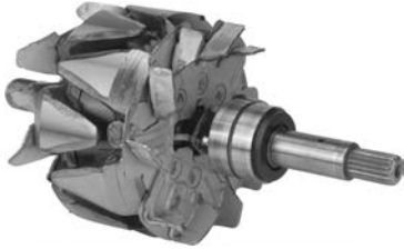
235774 Rotor
