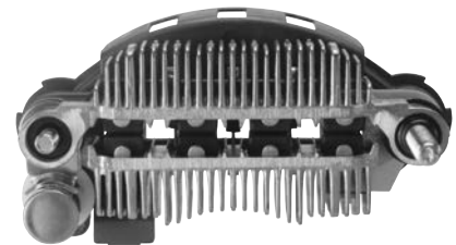
333056 Rectifier
