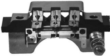
131699 Rectifier
