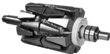
136462 Rotor
