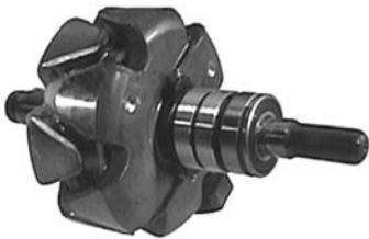
138150# Rotor
