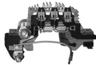
132938 Rectifier
