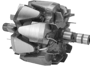
232198 Rotor
