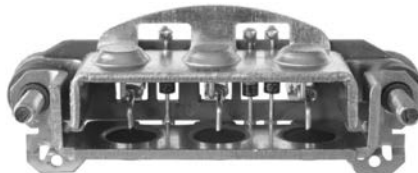
131543 Rectifier
